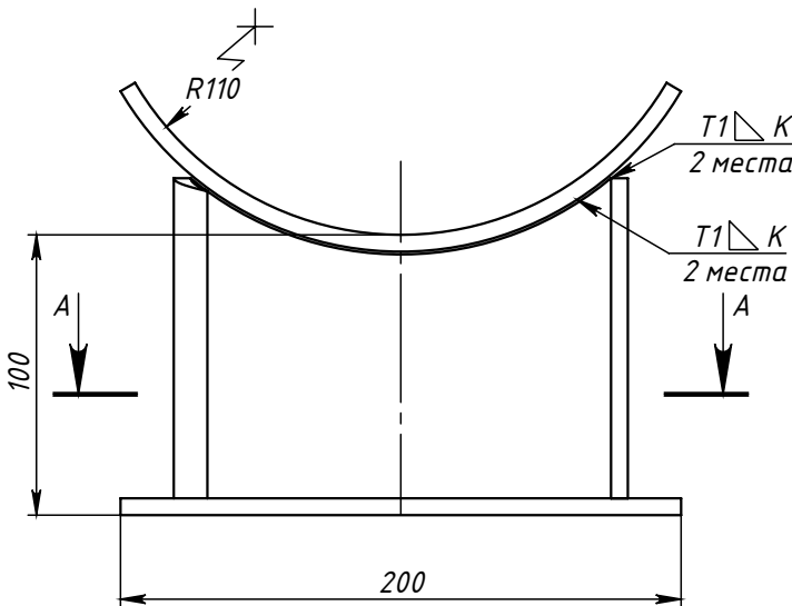
Поз.3 (Ложемент)
